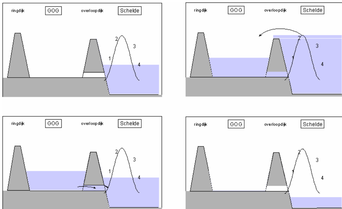
Figuur 7: Principe van de werking van een gecontroleerd overstromingsgebied (GOG)
