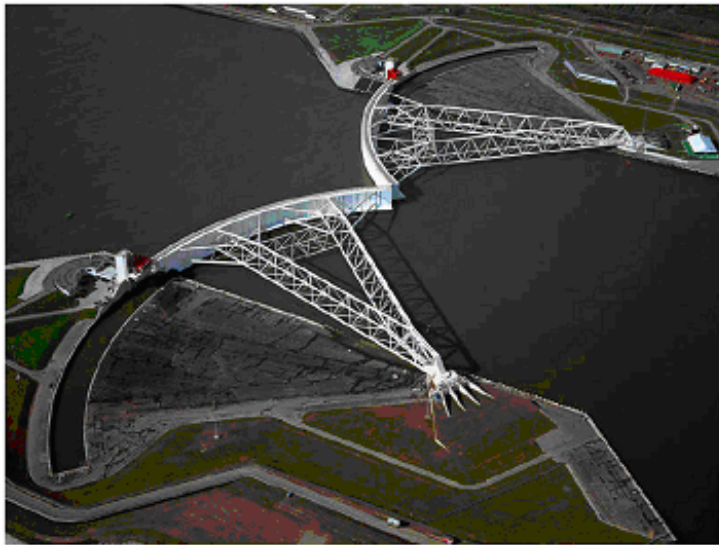
Figuur 9: Stormvloedkering van het type "nieuwe waterweg"
