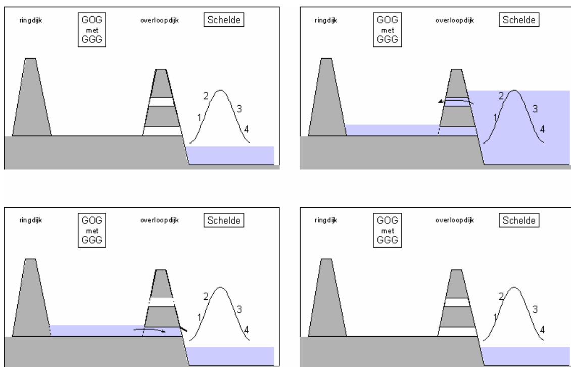
Figuur 8: Principe van de werking van een gebied met gereduceerd getij (GGG)
